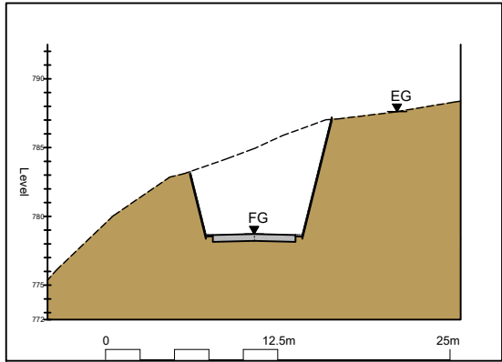
Section 10-A 1:500 @ A3 2.27
