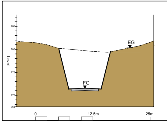
Section 10-D 1:500 @ A3 2.27
