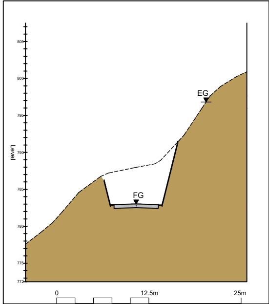
Section 10-C 1:500 @ A3 2.27
