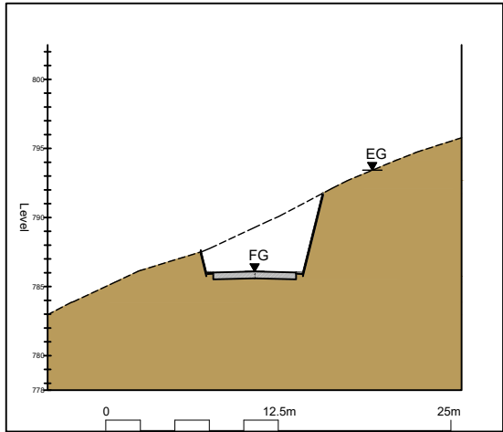
Section 10-B 1:500 @ A3 2.27
