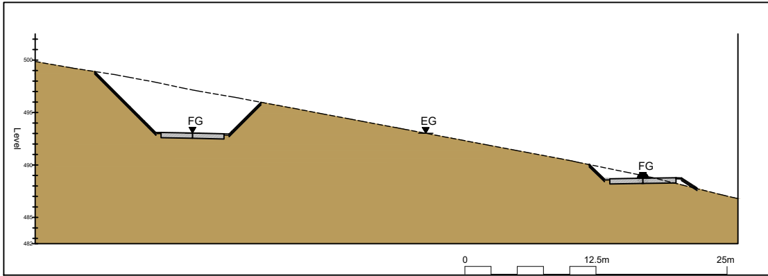
Section 3-A 1:500 @ A3 2.27
